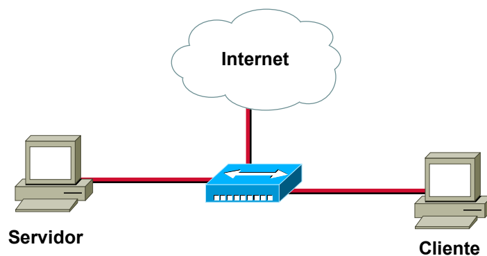
Figura 29. Esquema lógico experiencia 5
