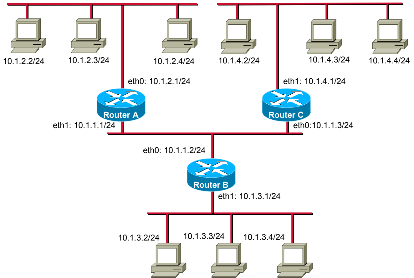
Figura 10. Enrutamiento IP
