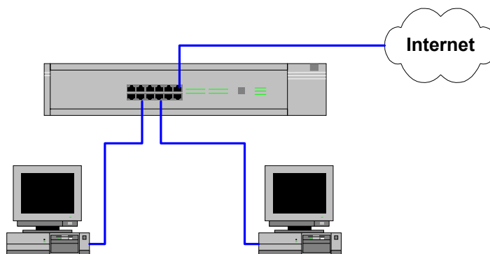
Figura 26. Esquema físico experiencia 3
