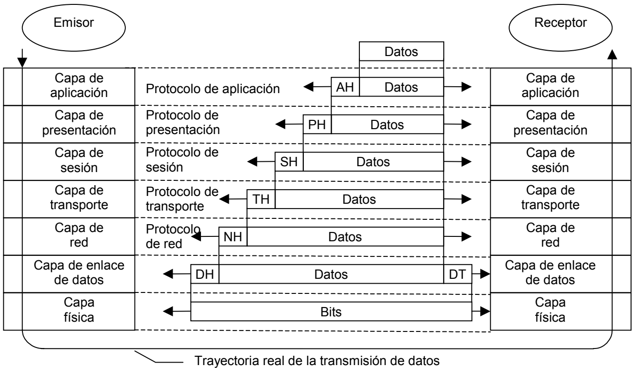
Figura 7. Ejemplo de uso del modelo OSI. Algunos encabezados pueden ser nulos
