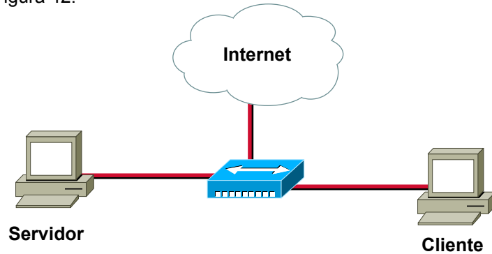
Figura 55. Esquema lógico experiencia 5
