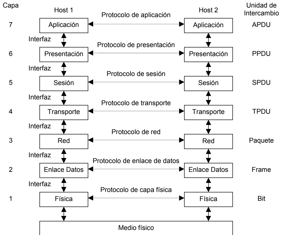
Figura 6. El modelo de referencia OSI
