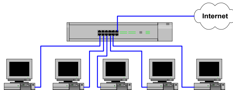
Figura 21. Esquema lógico del laboratorio 1
