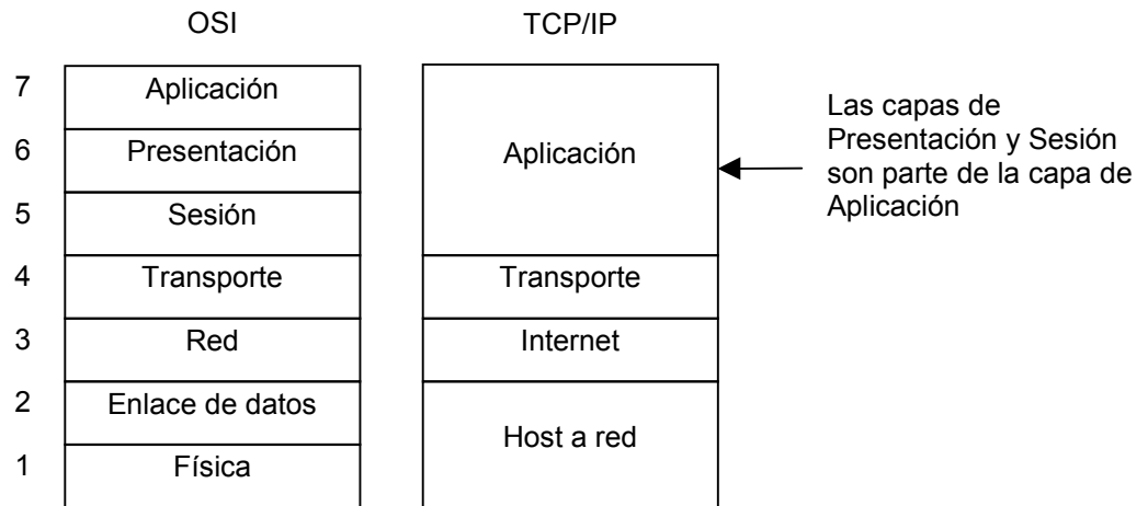
Figura 8. Las capas del modelo de referencia TCP/IP, comparadas con el modelo de referencia OSI
