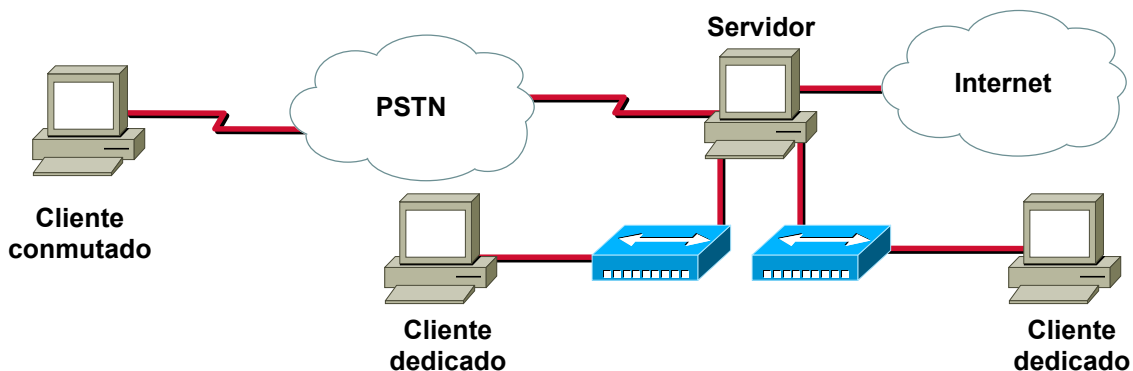
Figura 27. Esquema lógico del laboratorio 4
