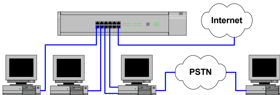
Figura 27. Esquema lógico del laboratorio 4
