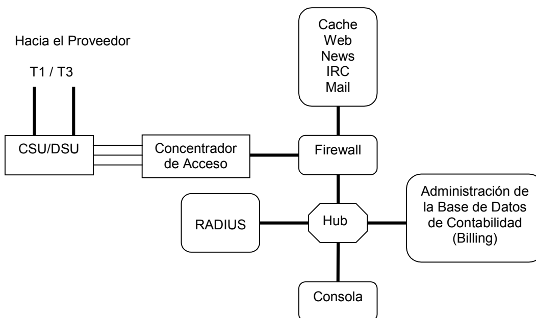
Figura 3: Diagrama en Bloques Mínimo de un ISP
