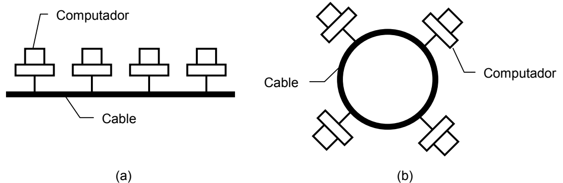
Figura 2. Topologías de redes LAN. (a) Bus. (b) Anillo
