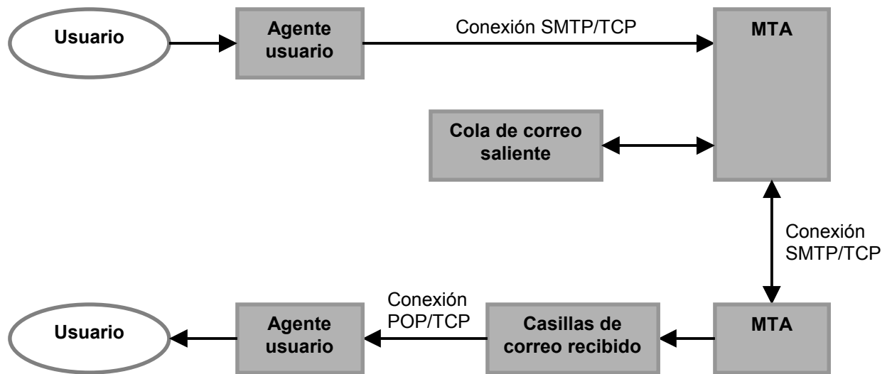
Figura 12. Esquema del correo electrónico Internet
