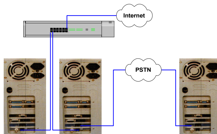
Figura 20. Esquema físico del laboratorio 0
