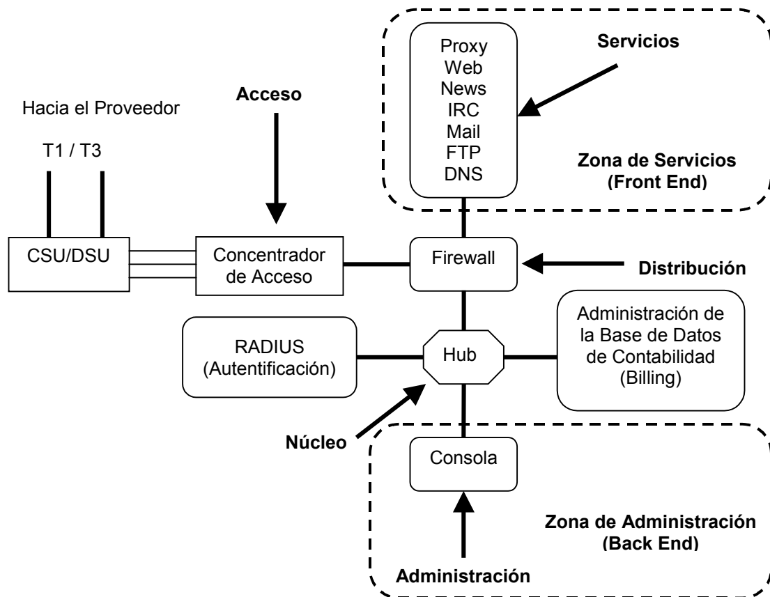
Figura 17. Estructura de un ISP mínimo
