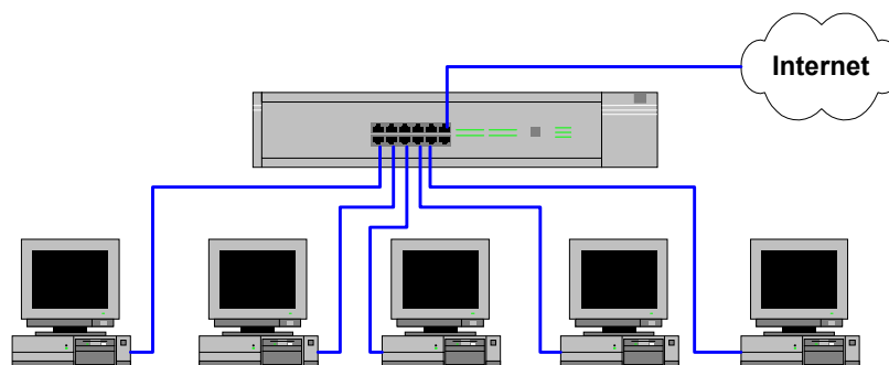
Figura 36. Esquema físico del laboratorio 1
