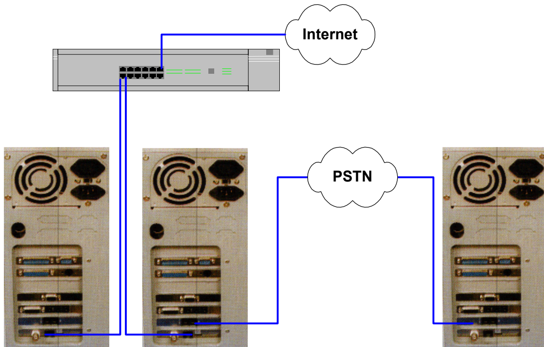
Figura 32. Esquema físico del laboratorio 0
