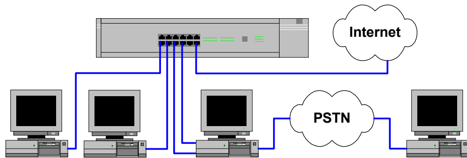
Figura 46. Esquema físico del laboratorio 4
