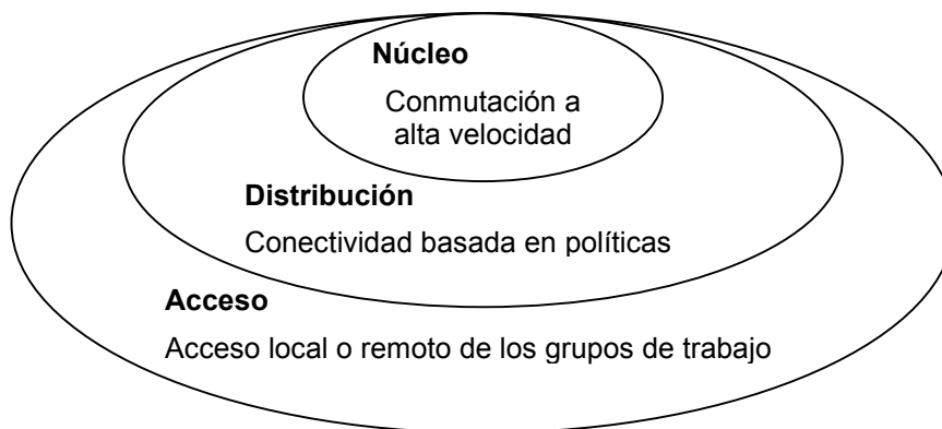
Figura 2: Modelo de Diseño Jerárquico de Redes
